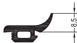
Уплотнение дверное № 3 (только для створок балконных дверей), SR
