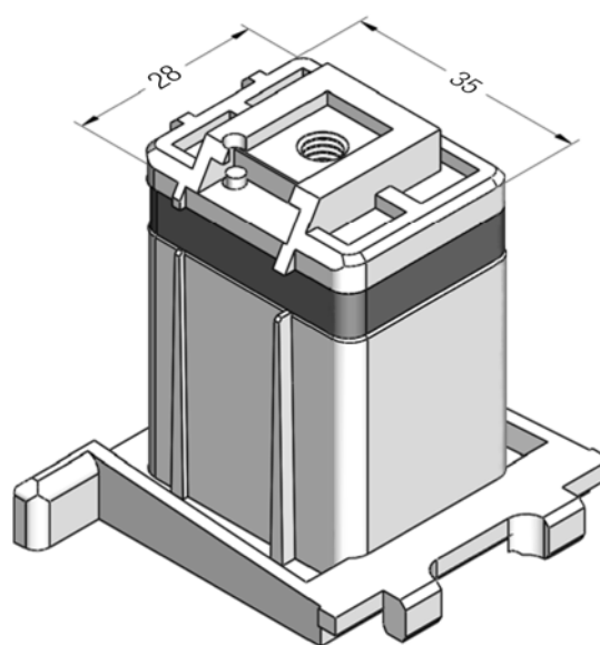
Механический соединитель импоста 86 BriD с уплотняющей манжетой,
